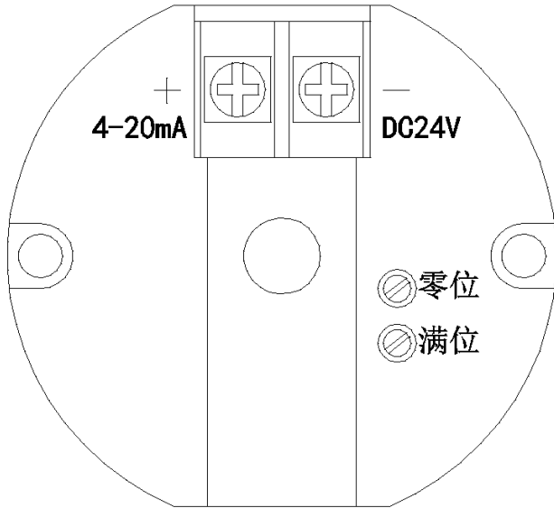
图一接线端子图
